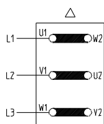
Connexion triangulaire 3 x 230 V, 50 Hz ou 220-240 V, 50 Hz
