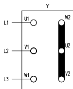
Conexión en estrella 3 x 400 V, 50 Hz resp. 380-420 V, 50 Hz
