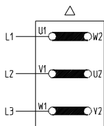
Conexión en triángulo 3 x 230 V, 50 Hz resp. 220-240 V, 50 Hz
