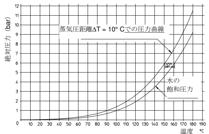
蒸気圧曲線
